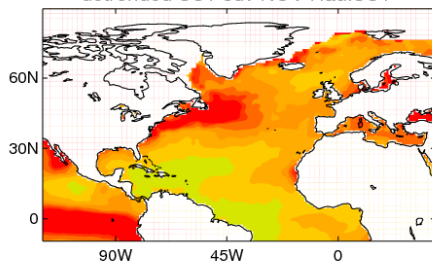
detrended SST sdv NOV HadISST
