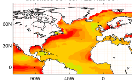
detrended SST sdv FEB HadISST
