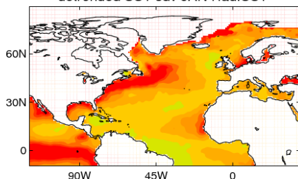
detrended SST sdv JAN HadISST
