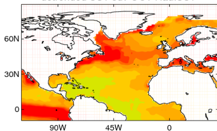
detrended SST sdv OCT HadISST
