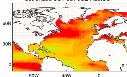
detrended SST sdv JUL HadISST
