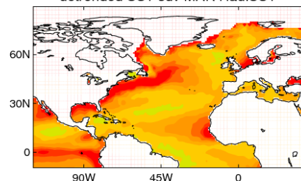
detrended SST sdv MAR HadISST
