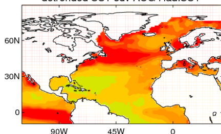
detrended SST sdv AUG HadISST
