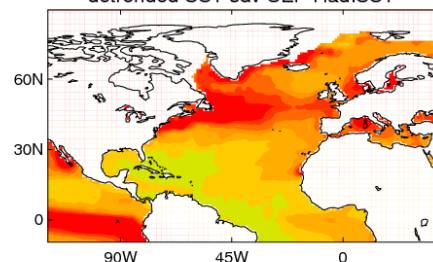
detrended SST sdv SEP HadISST
